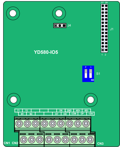
图 10-5 YD580-IO5 端子分布示意图
