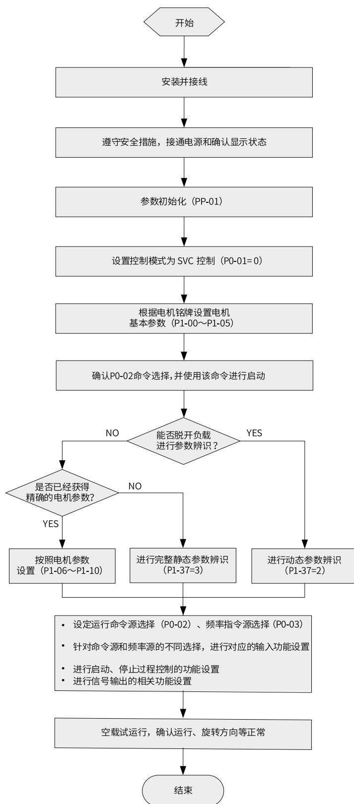
图 5-3 变频器调试流程图 (SVC)
