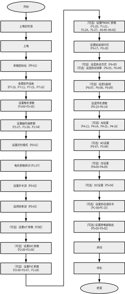
图15-1 基本调试流程图
