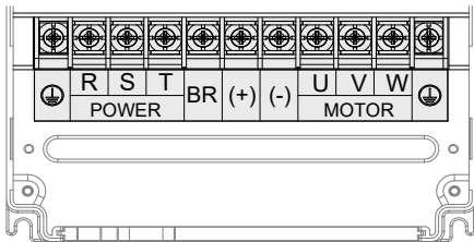
图 3-28 18.5kW~160kW 主回路端子分布图
