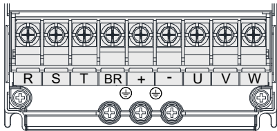
图 3-27 0.4kW~ 15kW 主回路端子分布图
