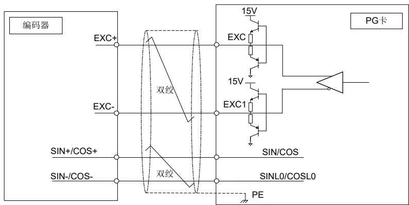
图 10-11 YD580-RZV 接口回路
