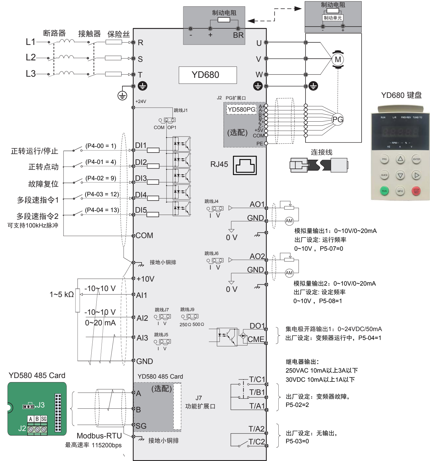
图 3-26 YD680 典型接线图
