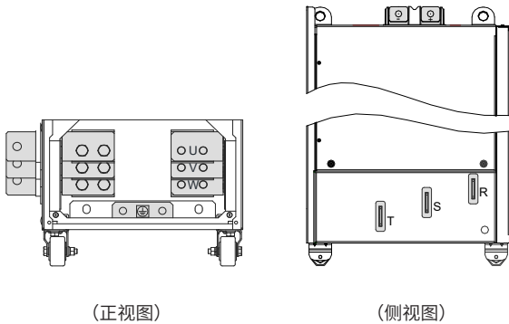
图 3-29 200kW~630kW 主回路端子分布图
