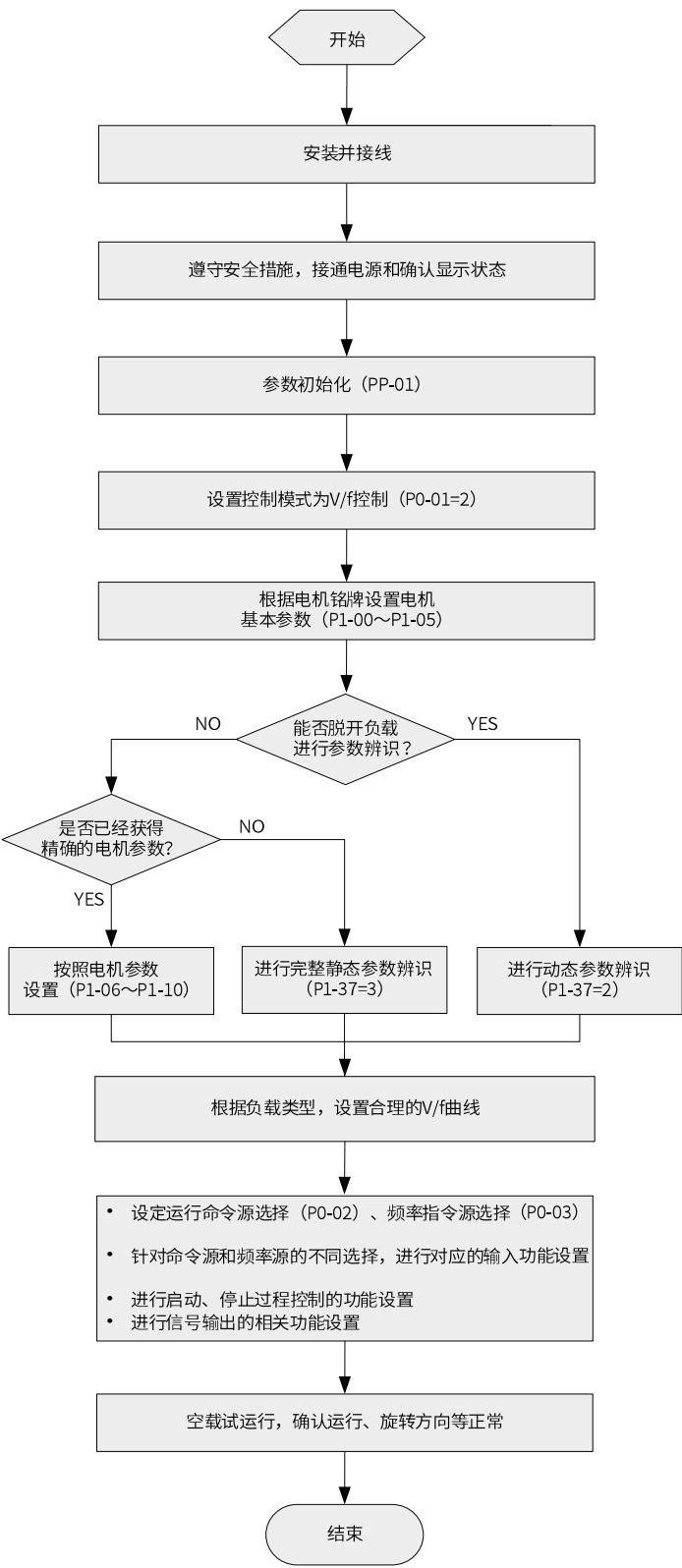
图 5-2 变频器调试流程图 (V/f控制)
