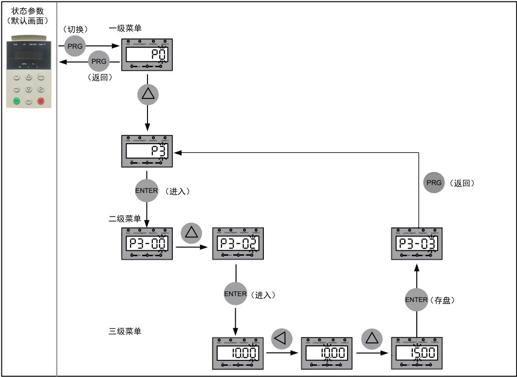
图4-3 参数修改操作示意图
