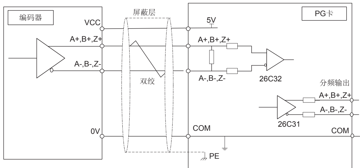
图 10-16 接口回路2
