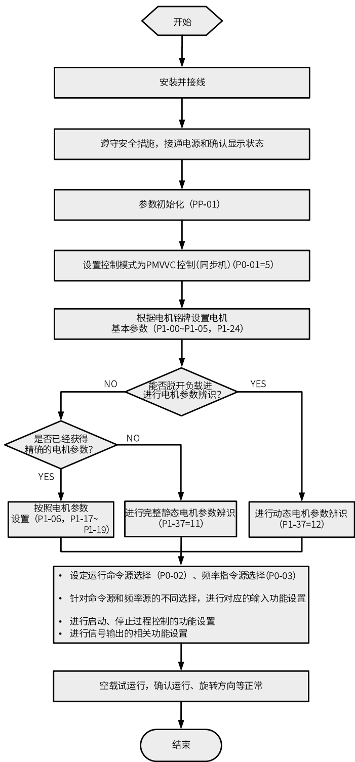
图 5-5 变频器调试流程图 (PMVVC控制)
