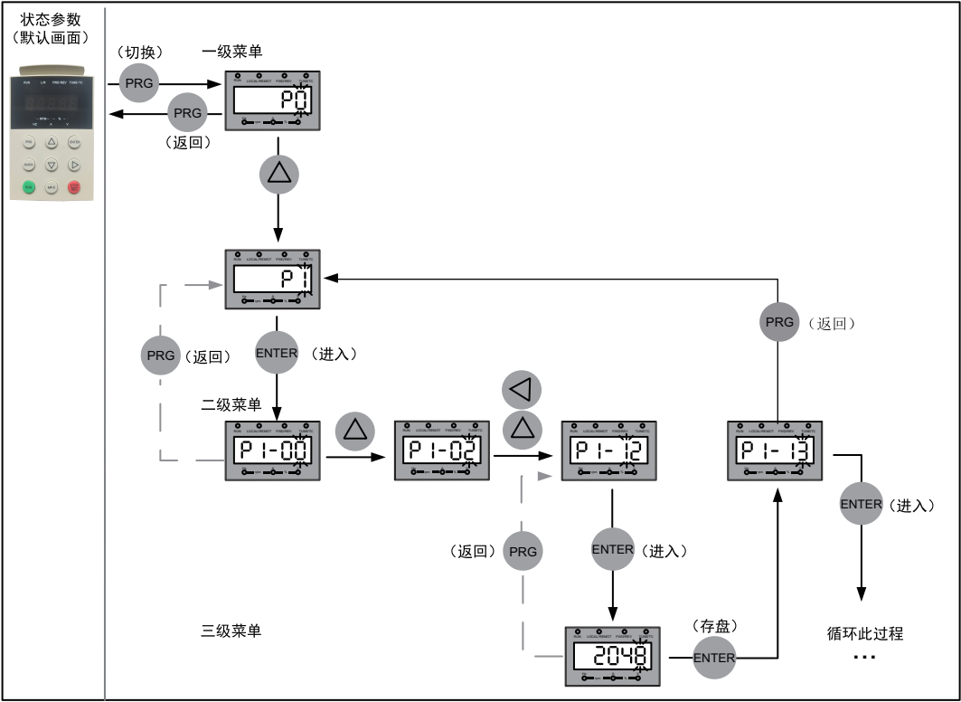
图4-4 参数查看操作示意图
