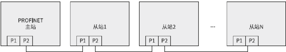
图2-3 总线型连接拓扑图
