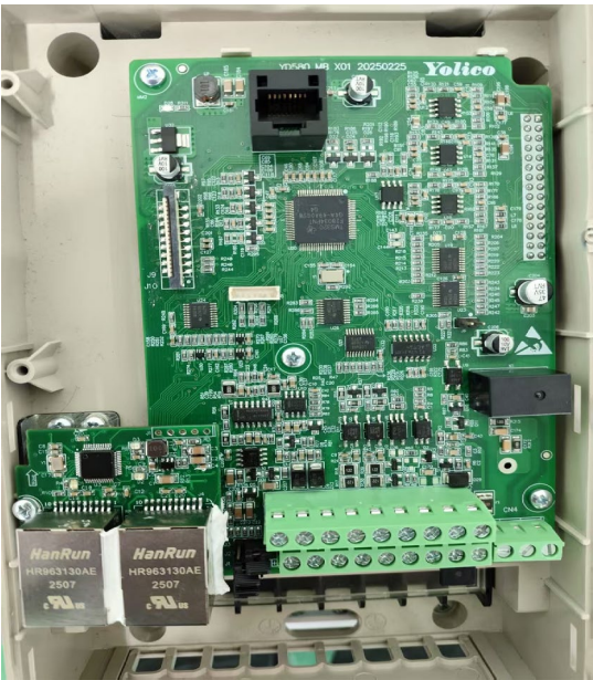
图2-1 YD580-PN卡安装示意图
