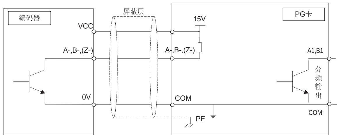
图 10-15 接口回路1
