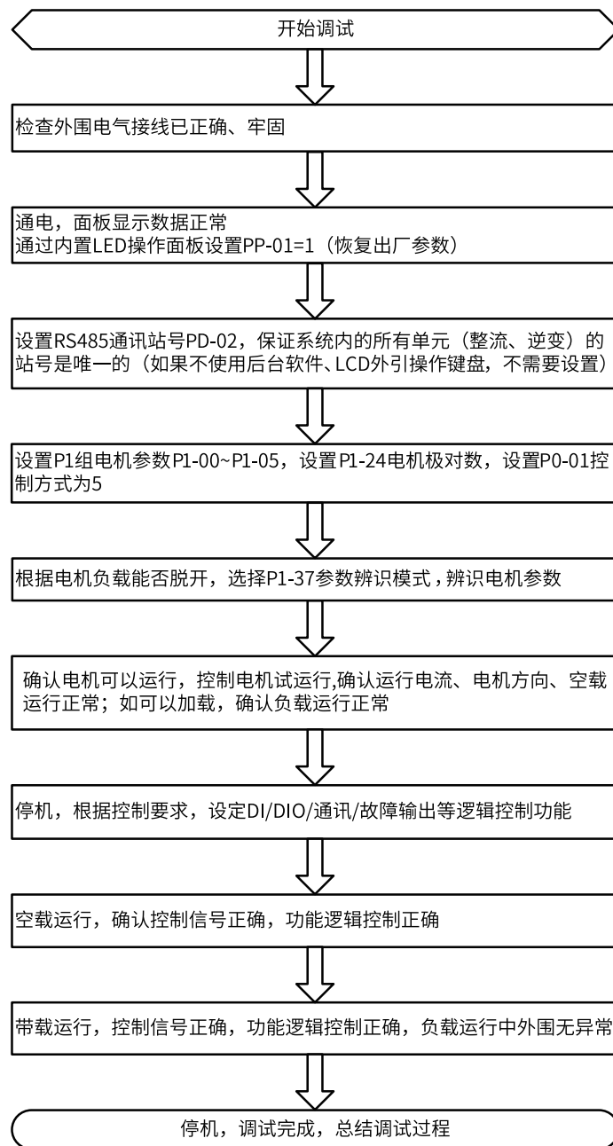
图 5-7 调试流程图
