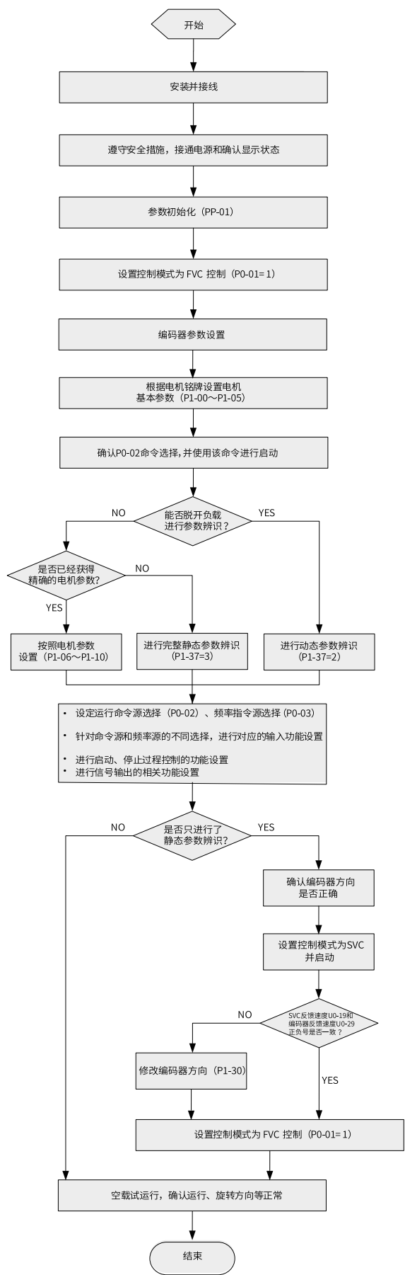
图 5-4 变频器调试流程图 (FVC)
