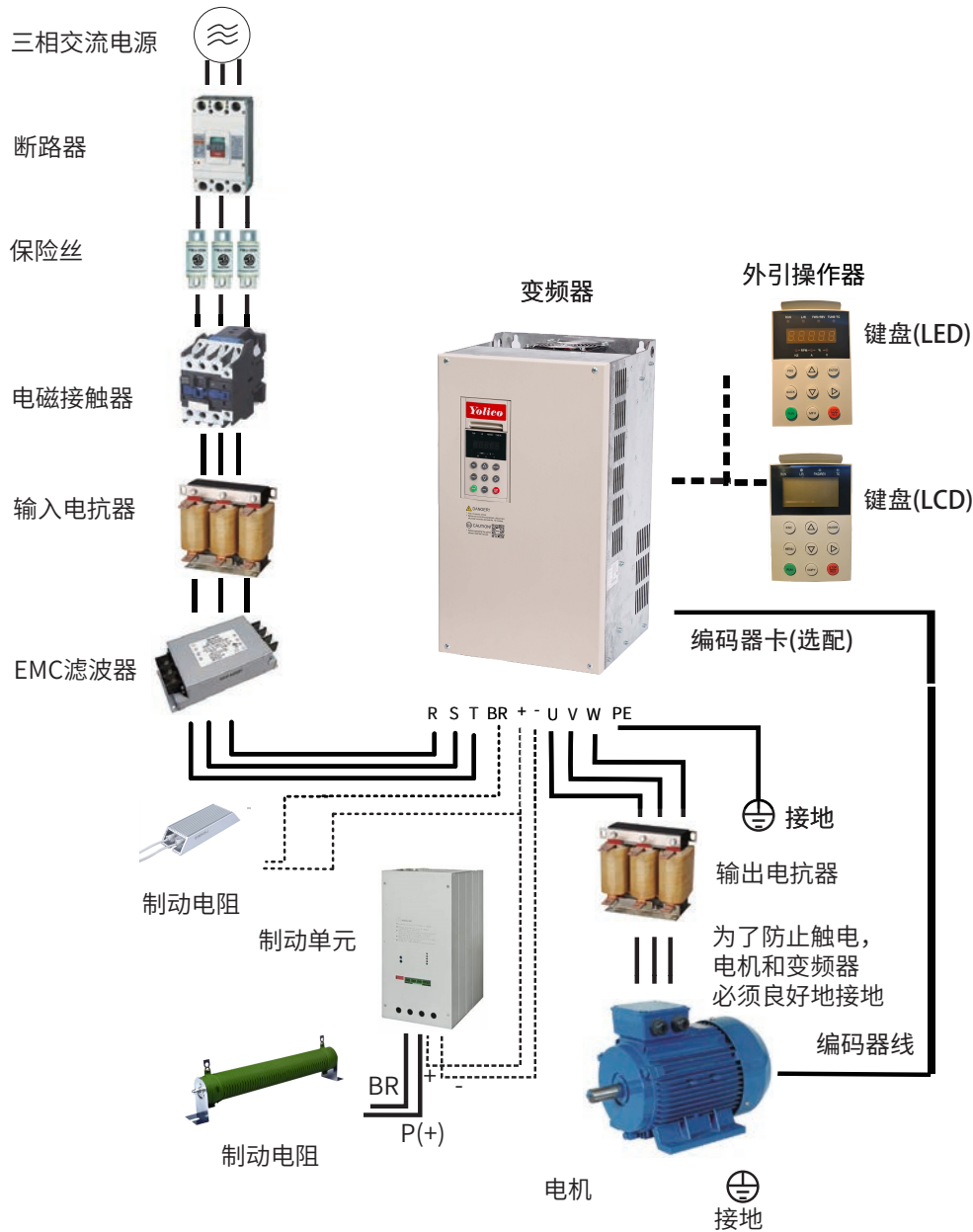
图 2-1 YD680 系列系统构成
